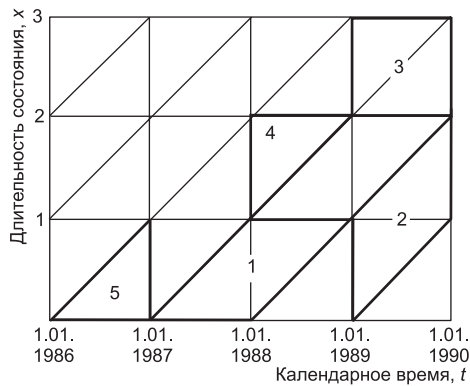
Рис. 1. Совокупности событий
