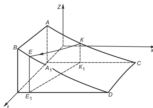
Рис. 1. «Поверхность Цейнера»
