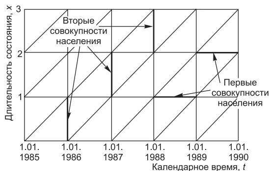
Рис. 2. Совокупности населения
