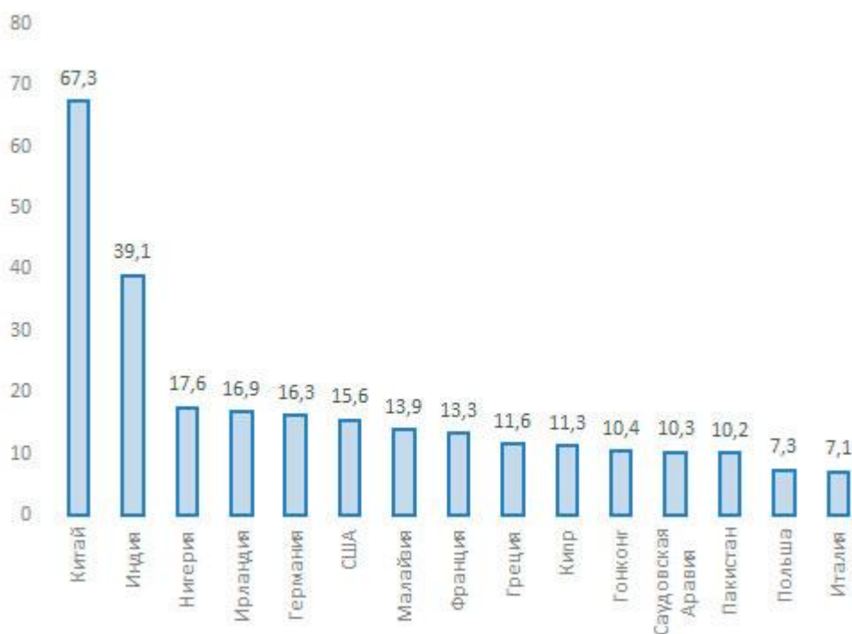
Рисунок 7. Образовательная миграция в Великобританию из 15 основных стран выхода иностранных студентов в 2010-11 учебном году, тыс. человек
