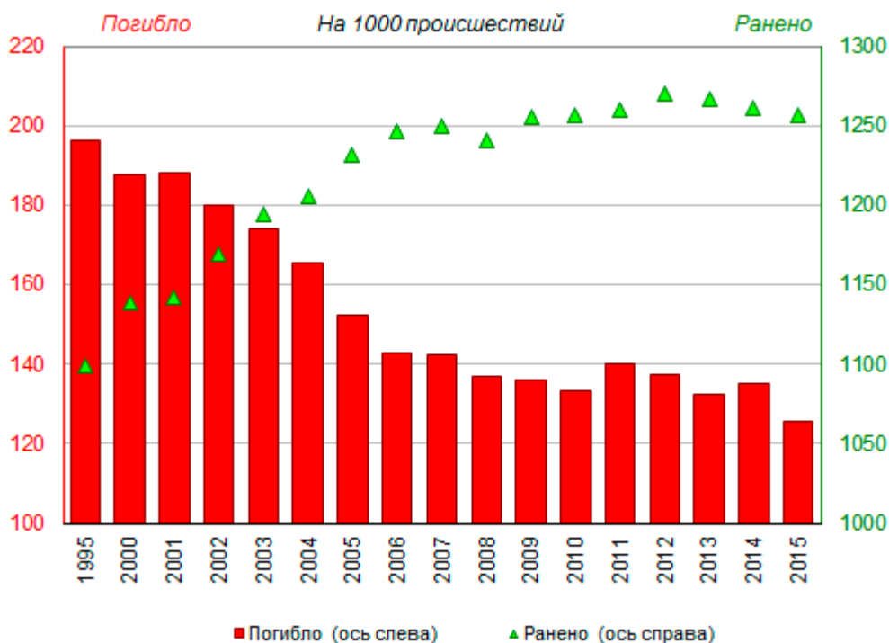
Рисунок 11. Число погибших (ось слева) и раненых (ось справа) на 1000 дорожно-транспортных происшествиях, 1995, 2000-2015 годы
